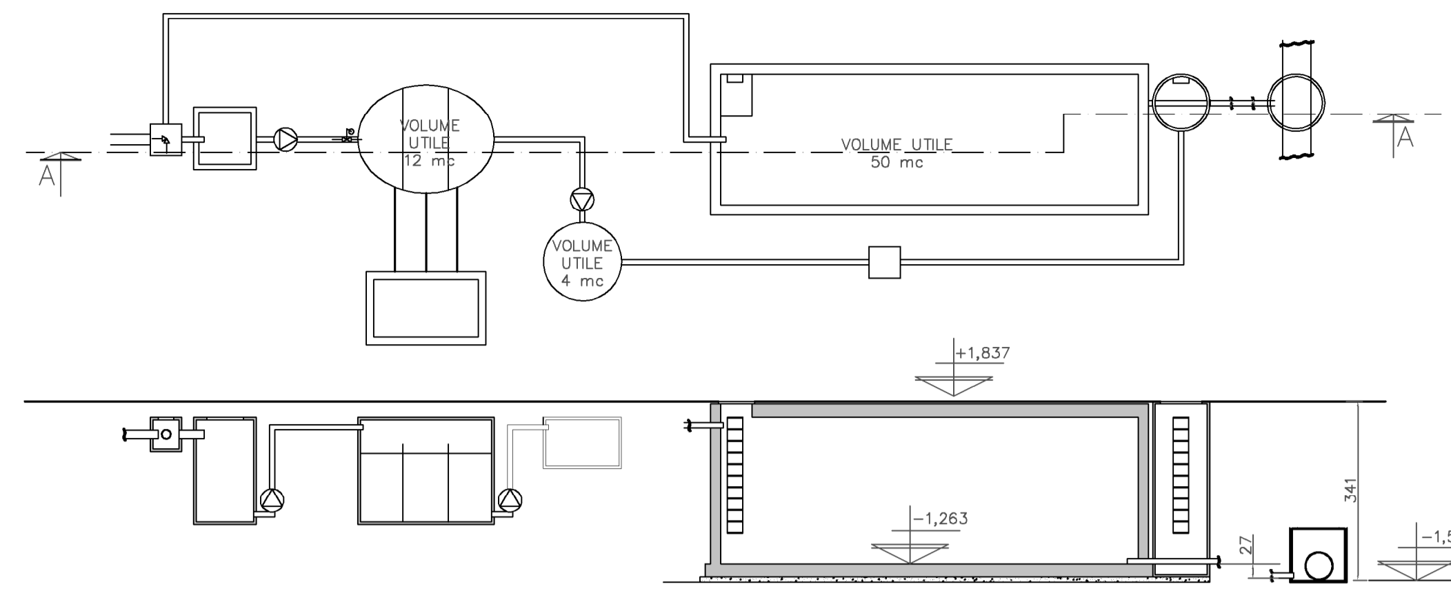
IMPIANTO VASCA DI LAMINAZIONE, PRIMA PIOGGIA E RACCOLTA ACQUE PIANTA E SEZIONE - scala 1:100
